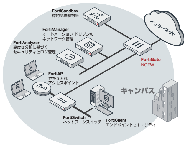
FortiGate 800D のキャンパスへの導入例 (NGFW)
