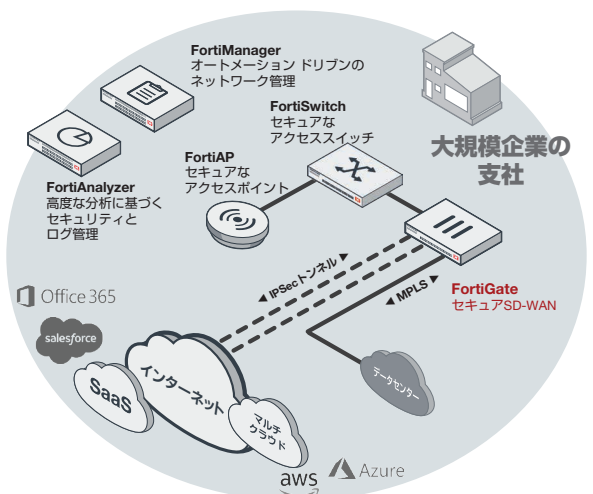
FortiGate 600E の大規模企業の支社への導入例 (セキュア SD-WAN)
