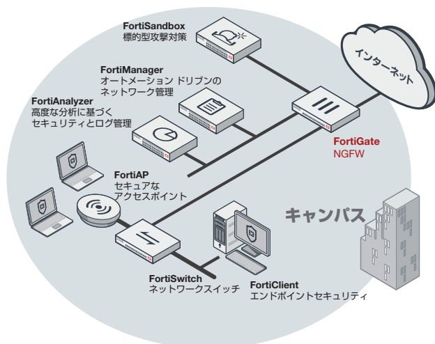
FortiGate 600E のキャンパスへの導入例 (NGFW)
