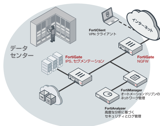
FortiGate 3700Dのデータセンターへの導入例 (NGFW、IPS、インテント ベースト セグメンテーション)
