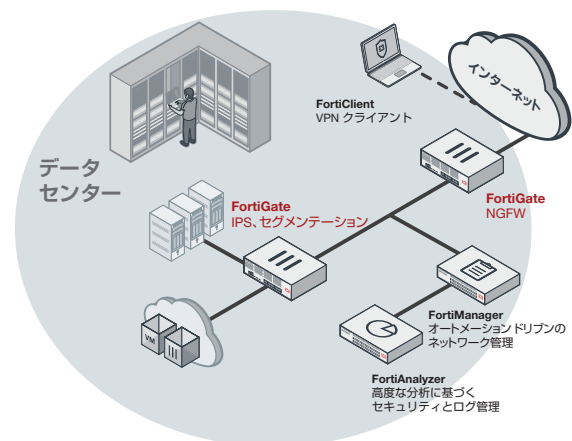
FortiGate 3200Dのデータセンターへの導入例 (NGFW、IPS、インテント ベースト セグメンテーション)
