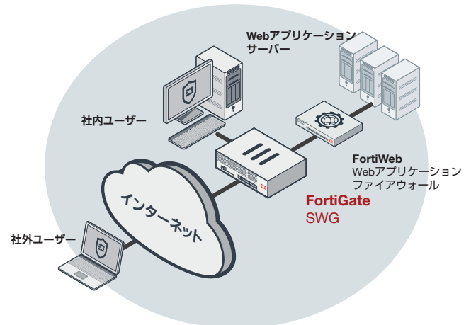
FortiGate 100E SWG の導入例
