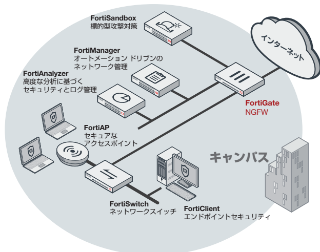
FortiGate 100E のキャンパスへの導入例 (NGFW)
